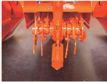
Verstelbare freesunit
