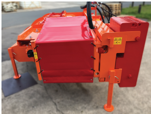
Gegengewichte für Balance in Arbeitsstellung
